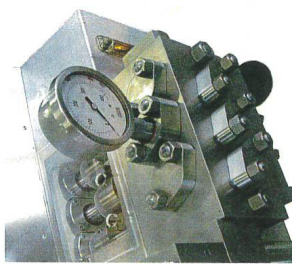
Dettaglio della testata di omogeneizzazione
